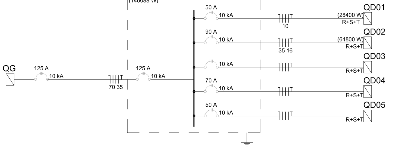
QUADRO GERAL DO PAVIMENTO (QGP) 5º PAVIMENTO (146088 W)
